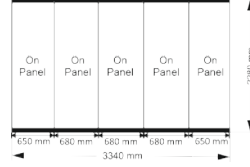
3X3 BASILABİLİR PANEL ÖLÇÜLERİ
