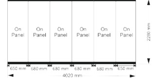
3X4 BASILABİLİR PANEL ÖLÇÜLERİ
